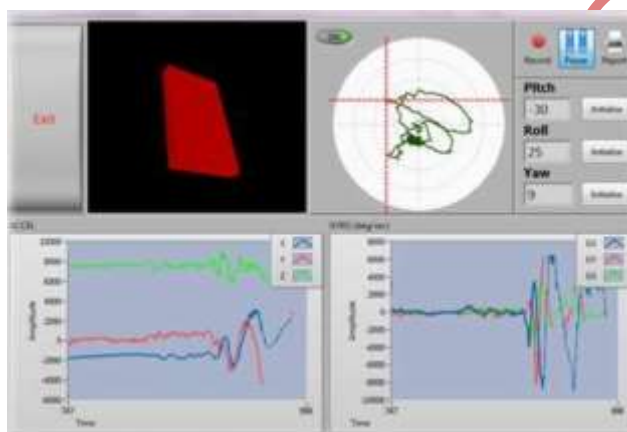
شکل ۱. نمایی از خروجی داده‌های مربوط به دستگاه ژيروسکوپ
